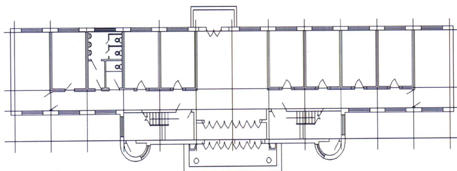
一层平面图
