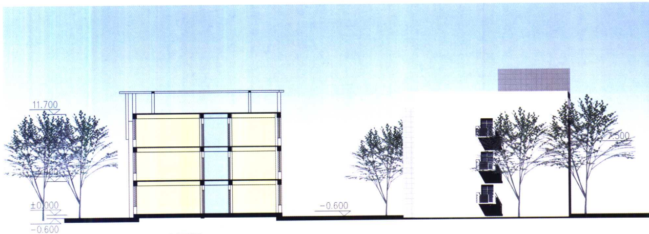
侧立面图
