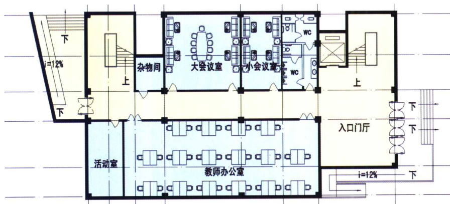
一层平面
