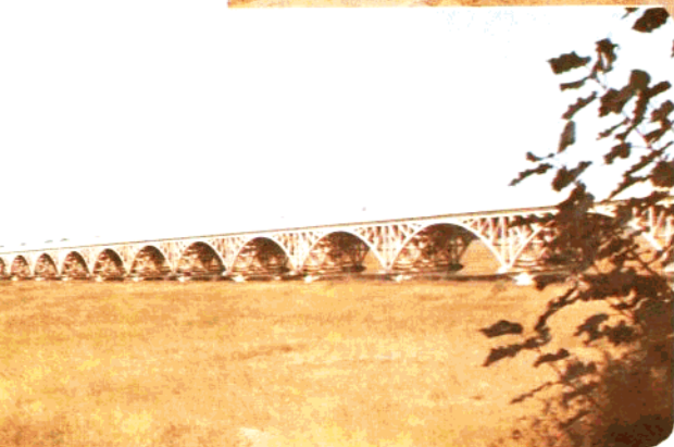
◀ 安新——高阳公路 同口钢筋混凝土桁架拱 特大桥
