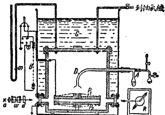
圖2. 密里根實驗裝置簡圖： a 是光源； w, d 是吸收熱射線的濾器。 P_1, P_2 是電容器， AD 是供應油滴的噴霧器； G 是油池（恆溫器）； B 是電池； m 是流體氣壓計； R 是檢流計。
