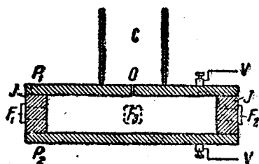
圖1. 密里根電容器的簡圖。
