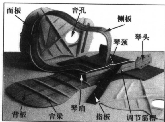
民谣吉他内部结构图
