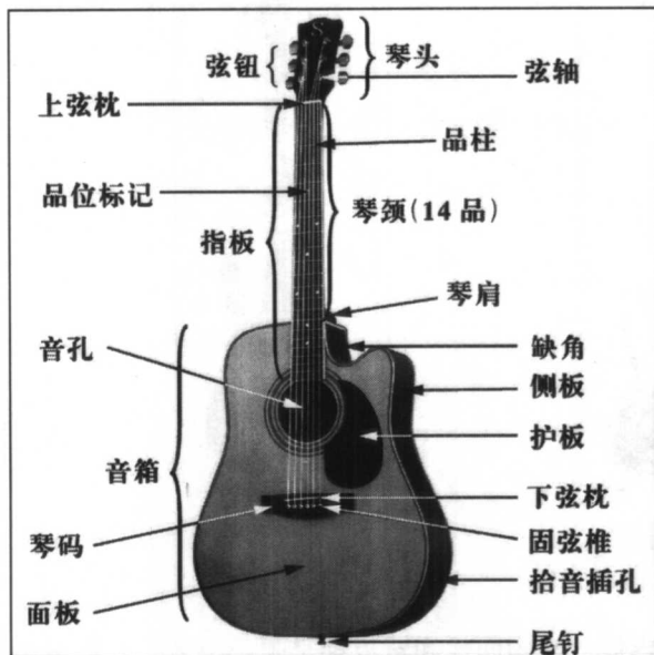
电箱缺角民谣吉他结构图
