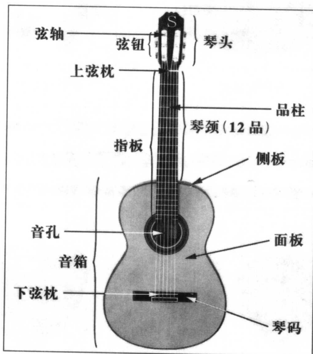
古典吉他结构图
