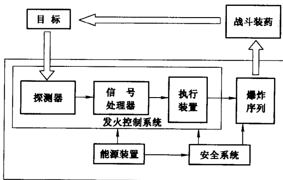
图 1-1 引信的基本组成及与目标和战斗部的关系
