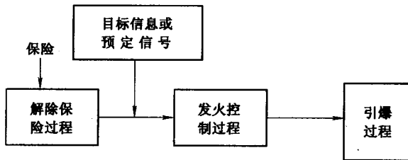
图 1-2 引信作用过程框图
