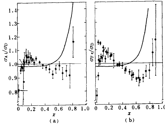
图 1.1.5 EMC 效应及每核子截面比值
