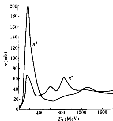
图 1.1.2 \pi^+ 和 \pi^- 被质子
