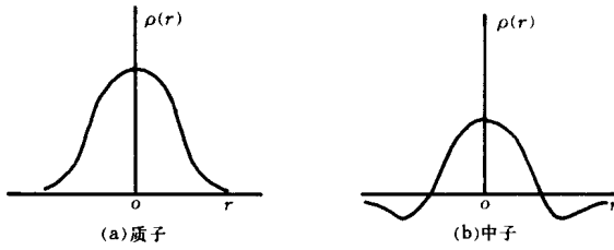
图 1.1.1 核子电荷分布示意图
