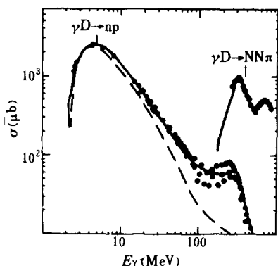
图 1.1.3 氘核的光致蜕变
