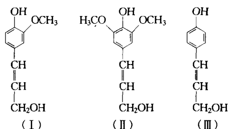
图 1-2 木质素不同类型的单体 I—松柏醇；II—芥子醇；III— \beta -茴香醇
