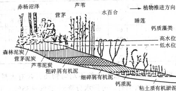
图 1-5 湖—沼演化中湖边泥炭和有机质淤泥形成示意图
