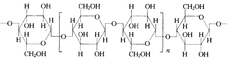
图 1-1 纤维素的分子结构
