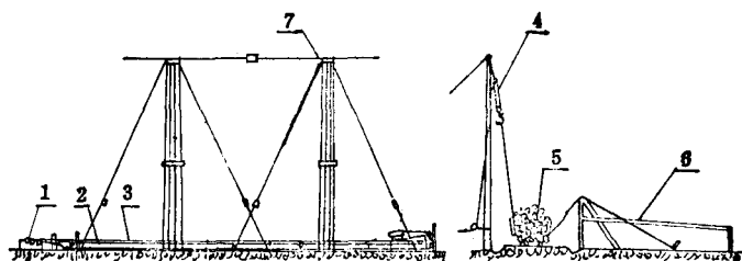
图 1 架杆兜卸机
