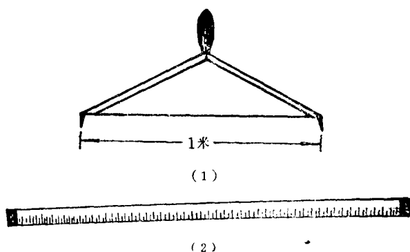
图6 1米弓形尺和2米竹尺 (1) 1米弓形尺 (2) 2米竹尺
