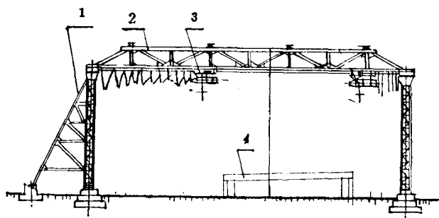
图3 固定卸车桥
