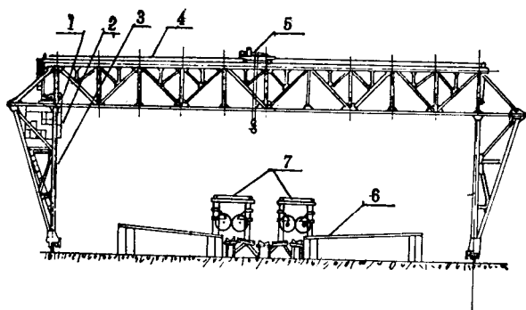
图5 龙门吊车
