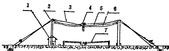
图 2 固定缆索起重机
