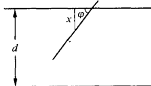
图 1.2.2 投针问题
