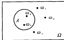
图 1.1.1 文氏图
