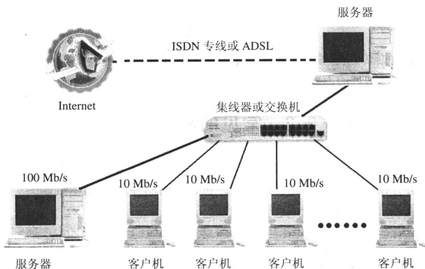
图 2.1 小型办公局域网
