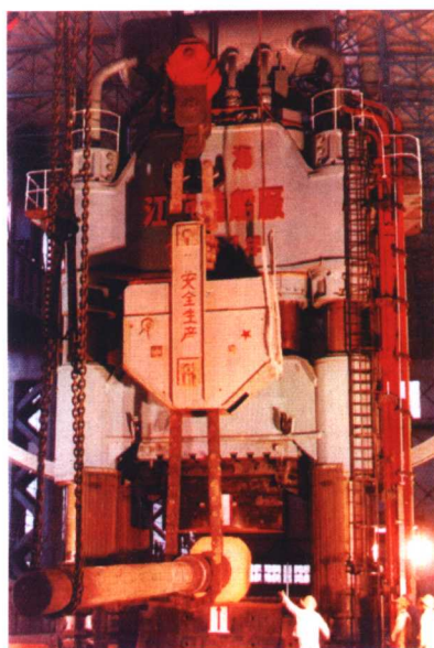
自力更生研制的万吨水压机
