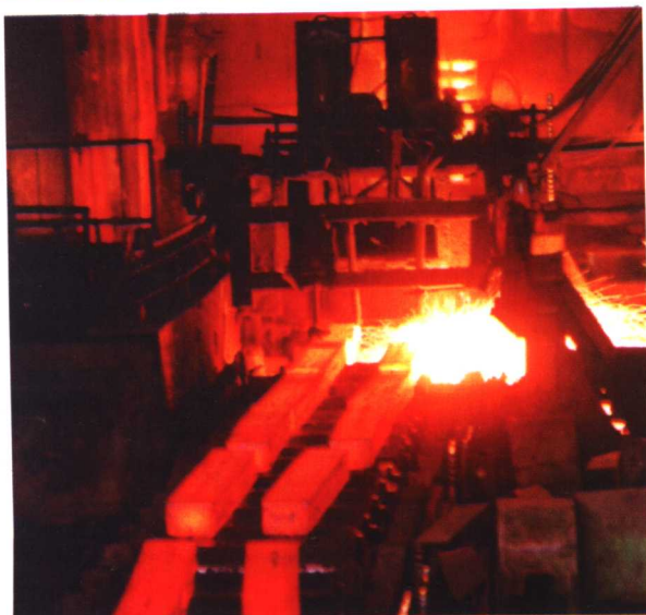
邯钢连铸车间
