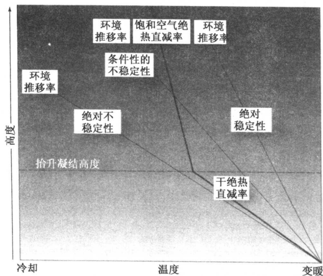
图4 温度直减率和稳定性
