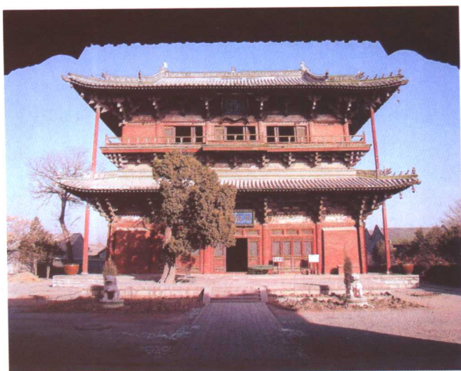
彩图 23 蓟县辽代独乐寺观音阁外观
