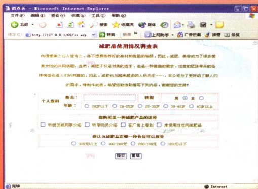
9-1_ 网上调查表
