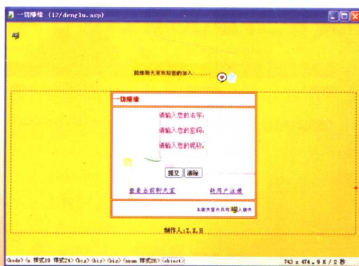
12-1_聊天室登录
