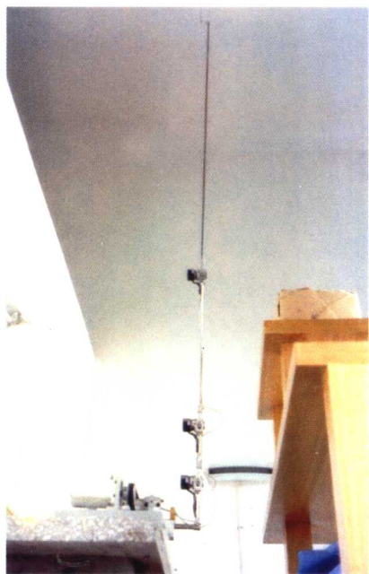
◀2002 年摄。世界首例 4 级倒立摆实物控制系统于 2002 年 8 月 11 日在数学系试验成功。
