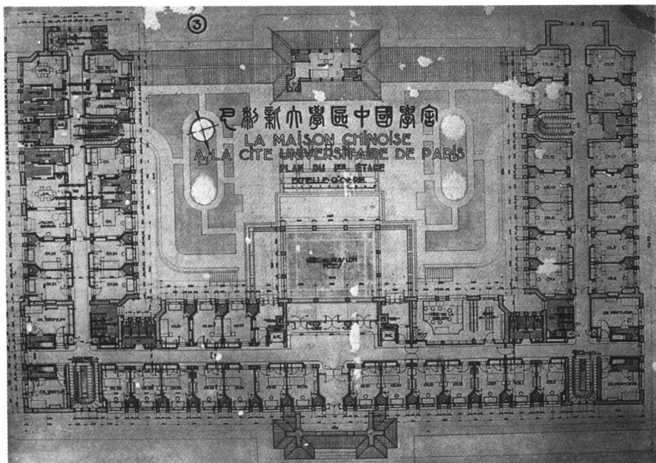
虞炳烈所作的“巴黎新大学区中国学舍”设计方案平面图
