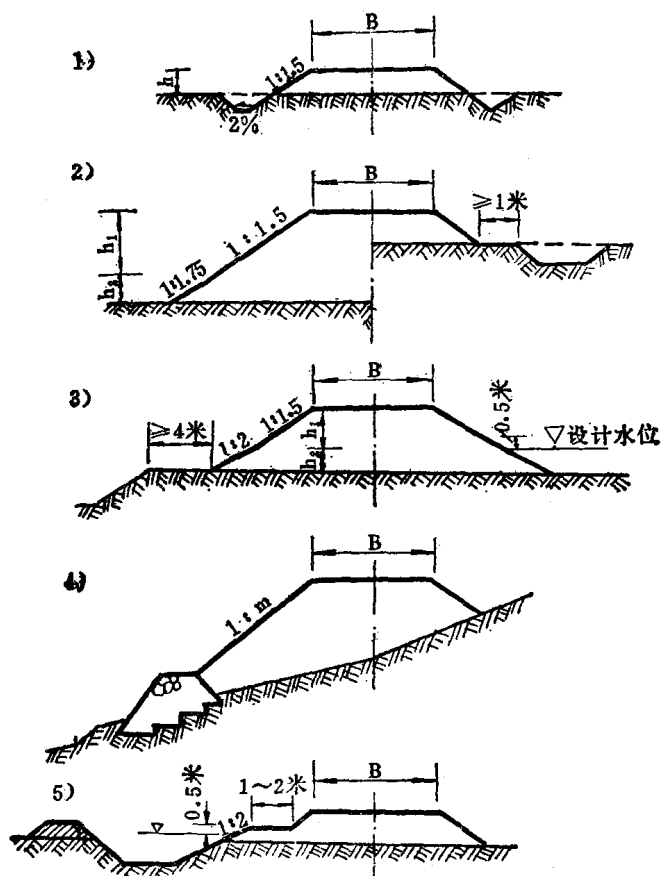
图1-1 填方路基典型断面图
