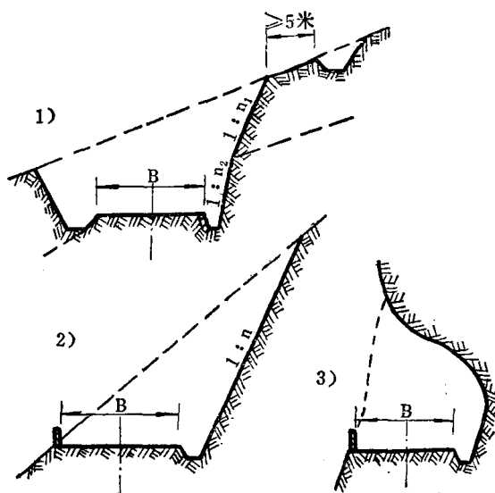
图1-2 挖方路基典型断面图
