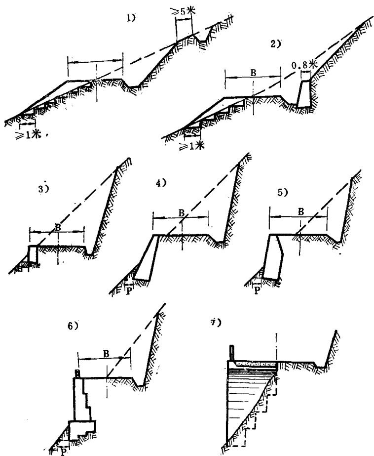
图1-3 半挖半填路基典型断面图
