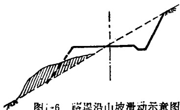
图1-6 路基沿山坡滑动示意图
