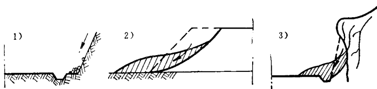
图1-5 路基边坡坍方示意图
