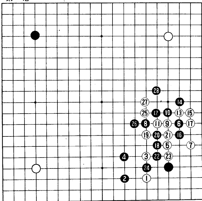
第一谱
