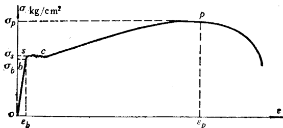
图 1-2 软钢的应力—应变曲线
