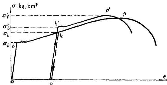
图 1-4 钢筋的冷拉
