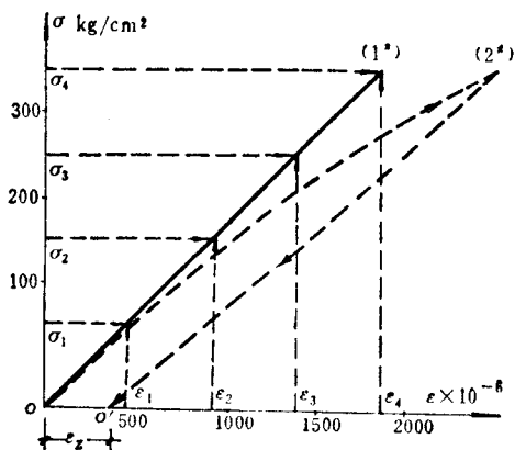
图 1-1 应力—应变曲线
