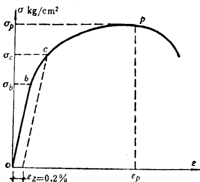
图 1-3 硬钢应变曲线
