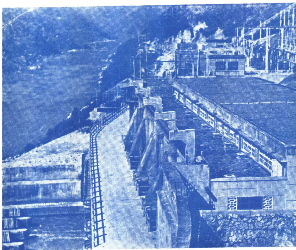
闽西南电力骨干工程之一华安水电厂——半掩式厂房全景
