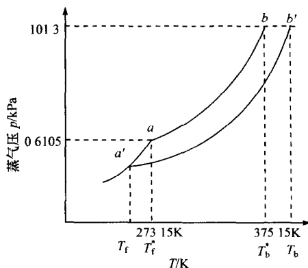
图 1-2 溶液沸点升高和凝固点下降
