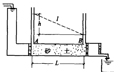
图 1-1 砂土渗透实验
