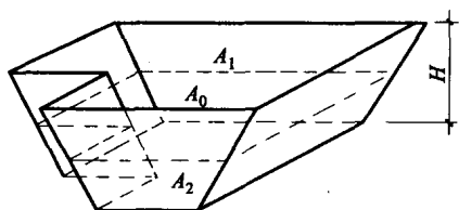
图 1-11 基坑土方量计算简图
