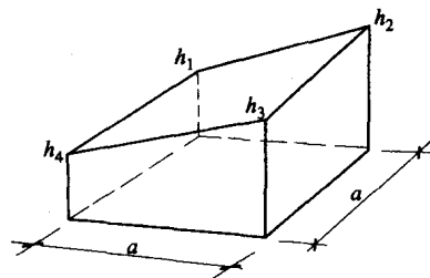
图 1-5 全挖或全填的方格
