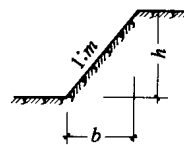
图 1-9 土方边坡示意图
