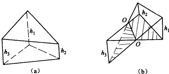
图 1-8 三角棱柱体法 (a)全挖或全填;(b)有挖有填
