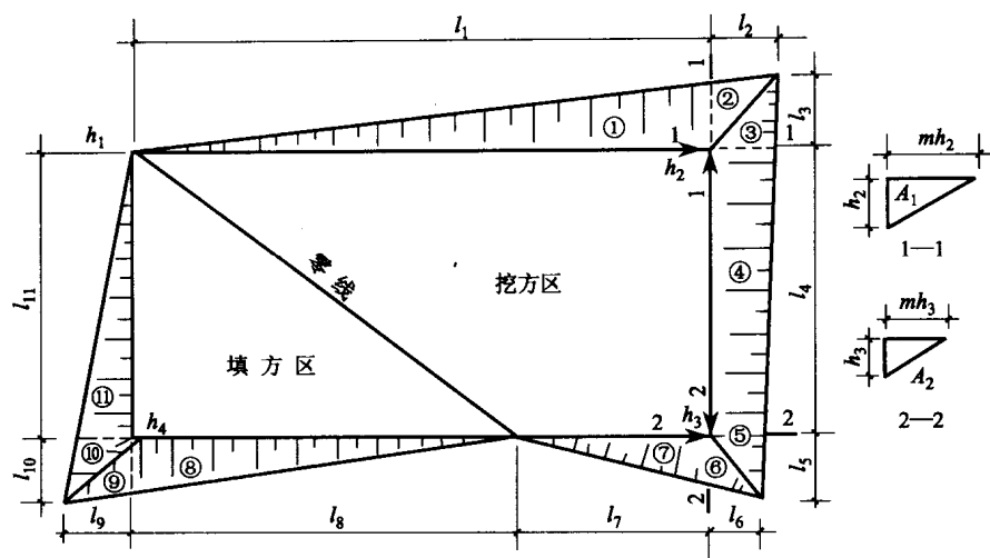
图 1-10 场地边坡平面图
