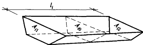
图 1-12 基槽土方量计算简图
