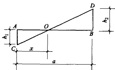
图 1-4 求零点的图解法
