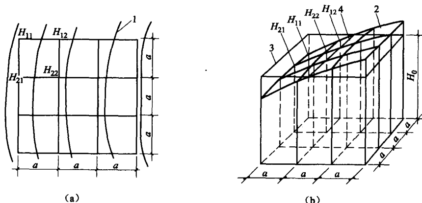
图 1-2 场地设计标高计算简图
