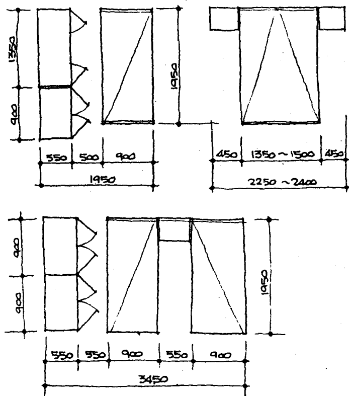
图 1—3 床与衣柜的平面尺寸
