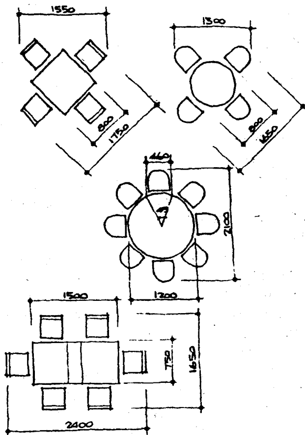
图 1-1 餐桌和椅的平面尺寸
