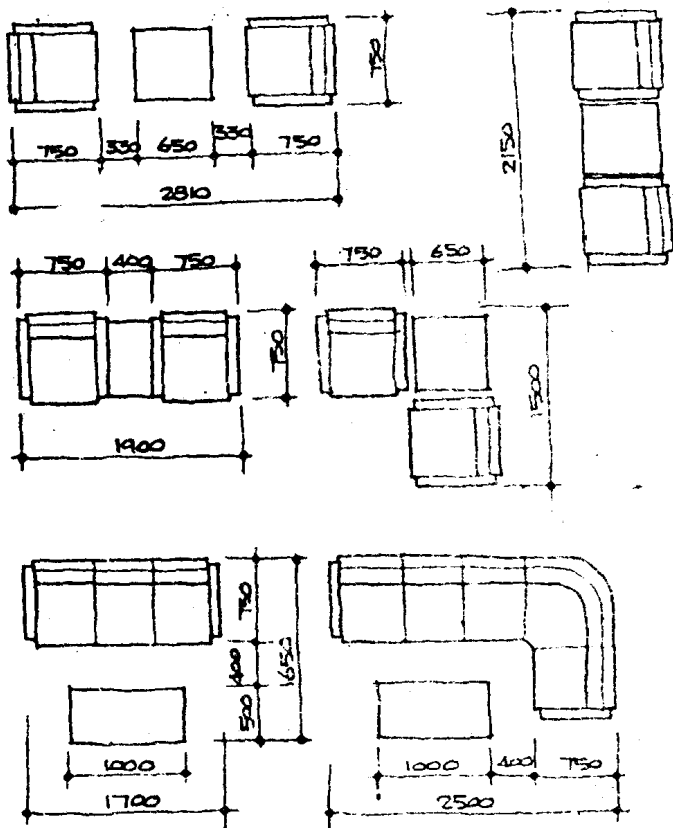
图1—2 沙发和茶几的平面尺寸
