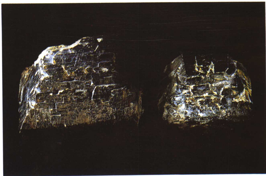
绿帘石(河北涉县。中国地质博物馆藏)
