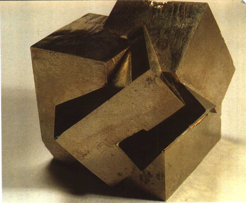
黄铁矿晶簇(西班牙。中国地质博物馆藏)
