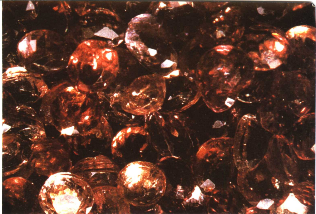
锆石戒面(据栾秉璪)
