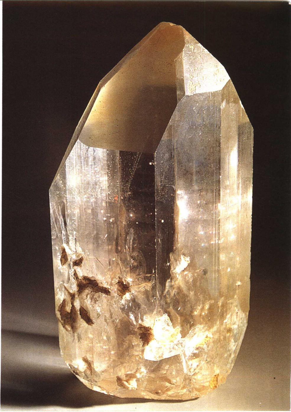
黄宝石(内蒙古。中国地质博物馆藏)
