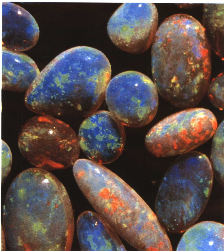
欧泊(澳大利亚)
