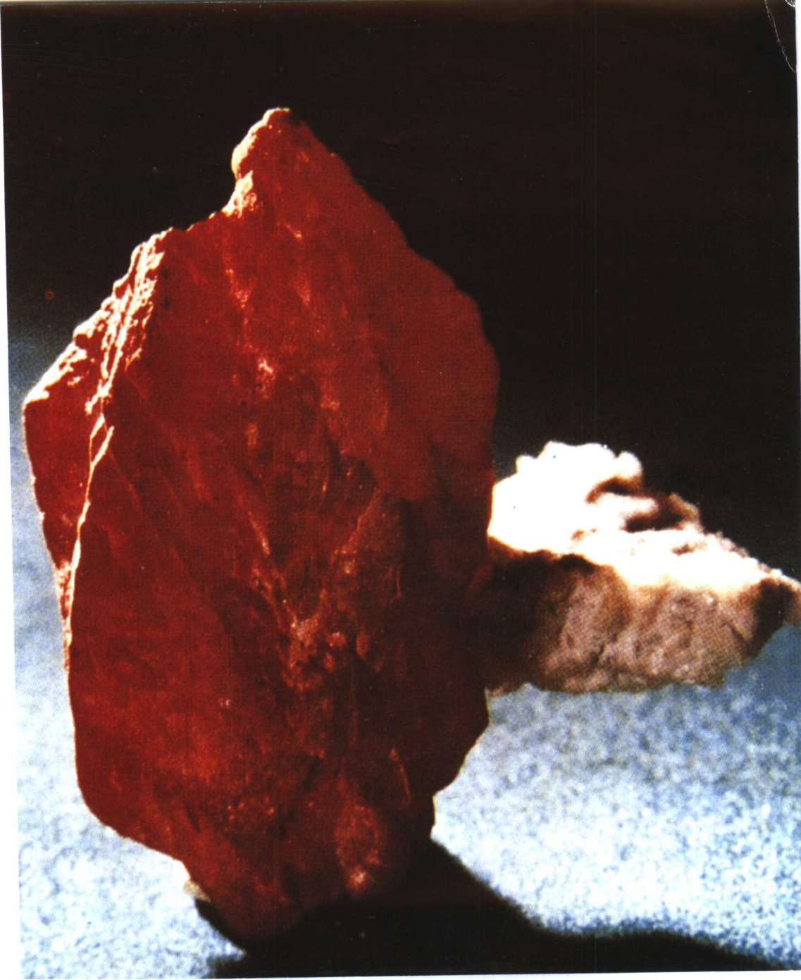
朱砂王(贵州万山汞矿区。 中国地质博物馆藏)
