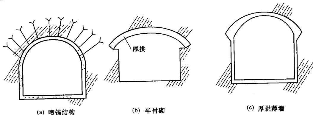
图 1.2 岩石中的地下空间建筑的结构型式
