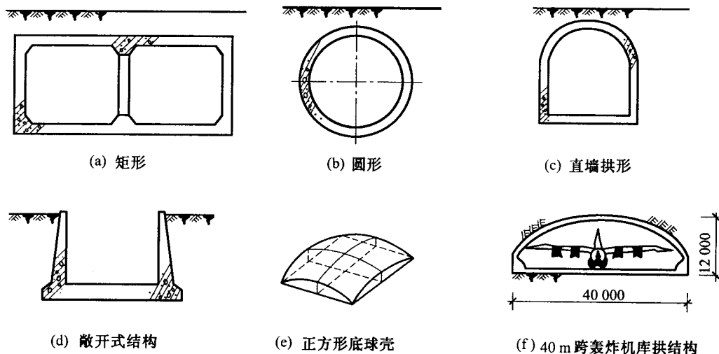
图 1.1 地下空间的结构型式
