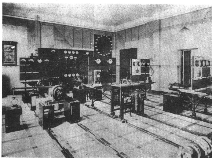
德文医工学堂的强电试验室
