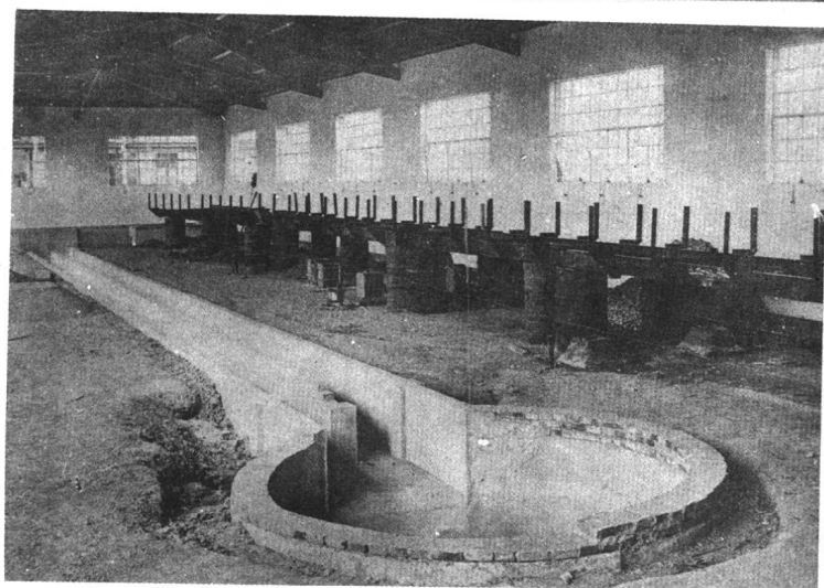
三十年代工学院水利试验场
