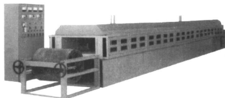
饼干生产线主设备：系列400~1000型隧道式远红外电烤炉 或系列400~1000型节能超导液炉
