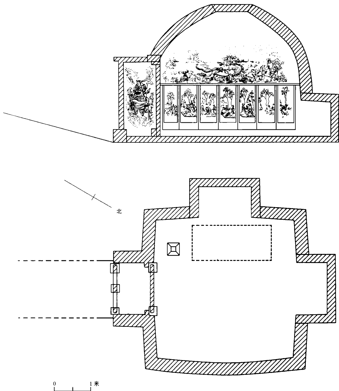
图二 崔芬墓平、纵剖面图
