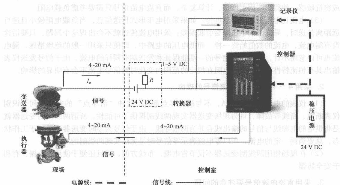
图 1.1 控制系统仪表之间的典型连接方式
