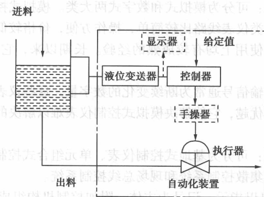
图 1 储罐液位自动控制系统
