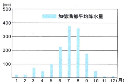
加德满都的降水量
