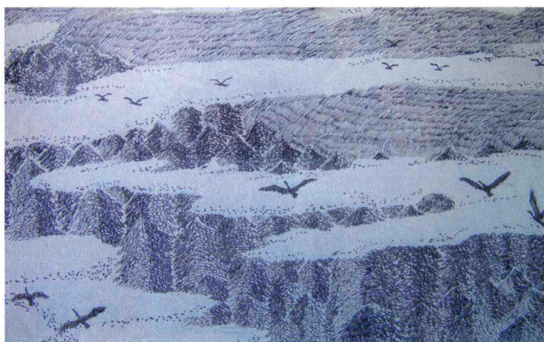
山林
