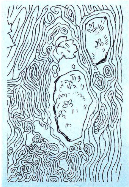
溪泉
