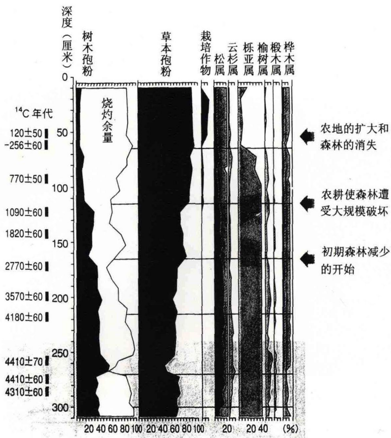
图四 内蒙古自治区卧龙泉的孢粉图 (安田喜宪等绘制)
