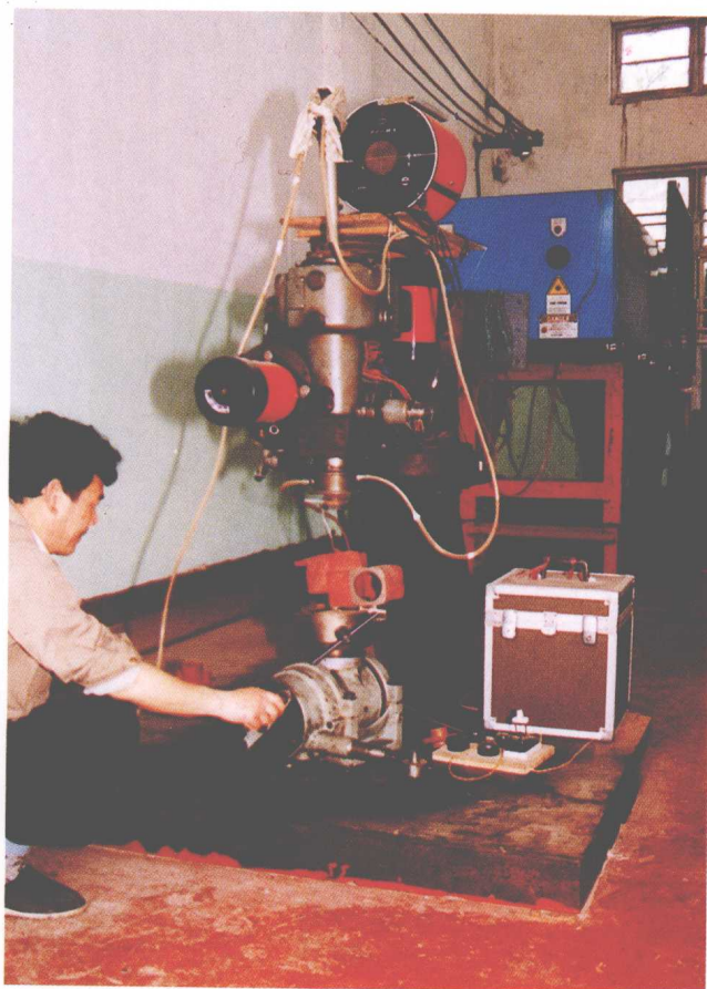
江西方向机厂采用激光热处理转向器壳体
