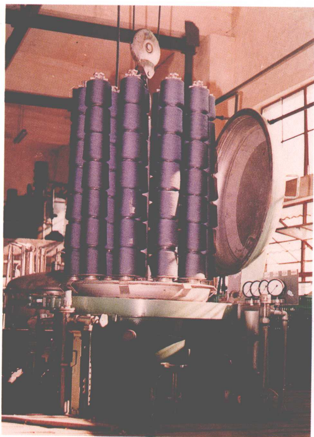
江西柴油机厂生产的MF245-100型筒子纱染色机， 1990年国家经委批准为替代进口产品
