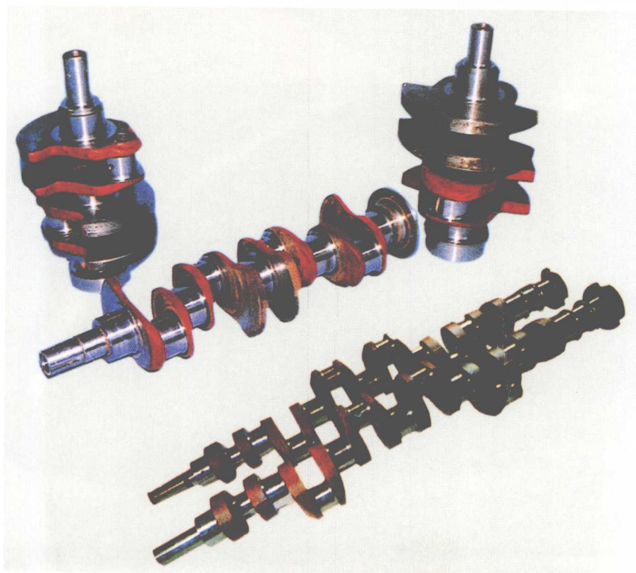
九江曲轴厂生产的 290、295、492Q、6160A 等各种机型柴油机、汽油机曲轴
