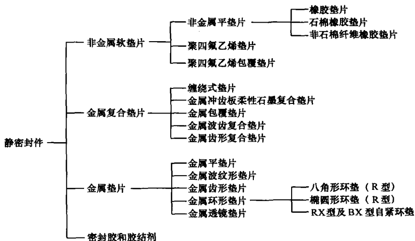
图 1-1 静密封件的分类
