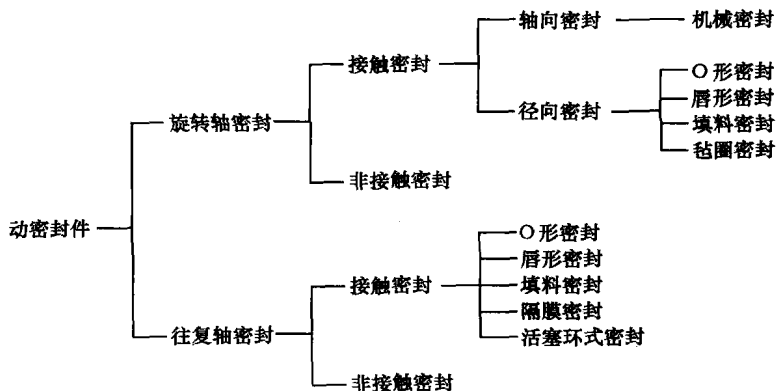
图 1-2 动密封件的分类
