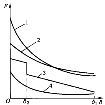
图 1-3 吸力特性与反力特性 1—直流吸力特性 2—交流吸力特性 3—反力特性 4—剩磁吸力特性
