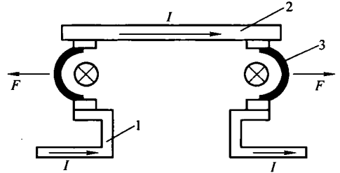
图 1-8 双断口电动力灭弧 1—静触头 2—动触头 3—电弧
