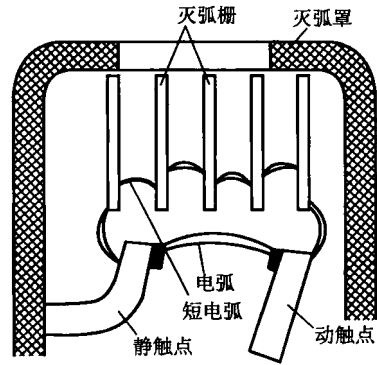
图 1-10 栅片灭弧装置
