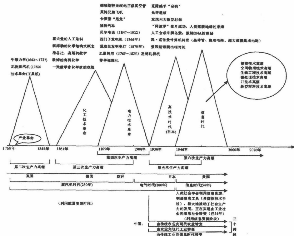
图3 1769~2010年人类社会生产力发展示意图
