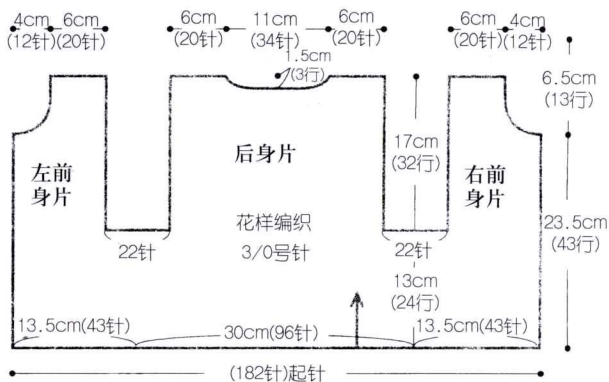
结构图
