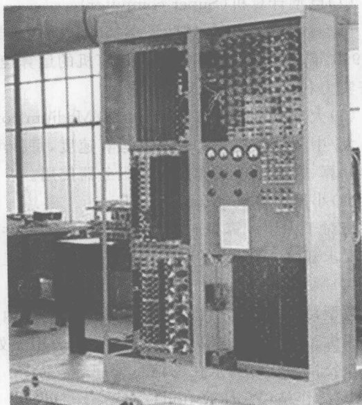
图 1-1 第一台电子计算机 ENIAC
