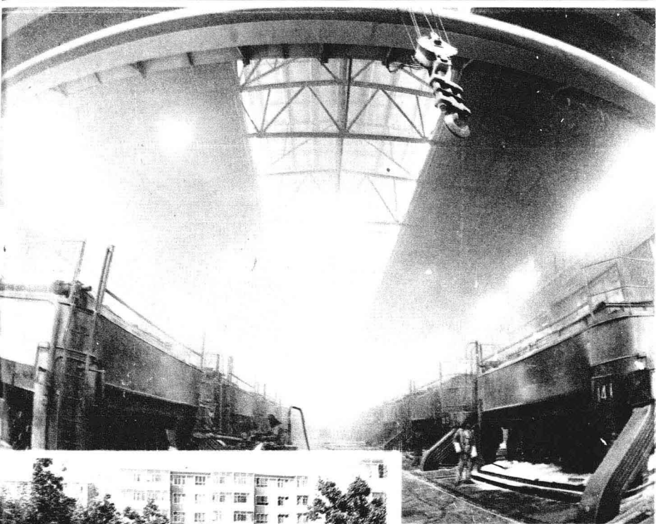
铝业公司冶炼厂电解车间
