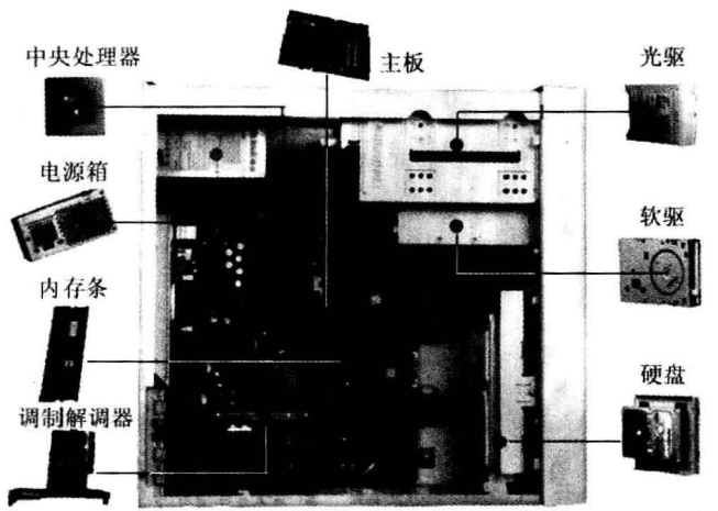
图 1-3 主机的基本组成
