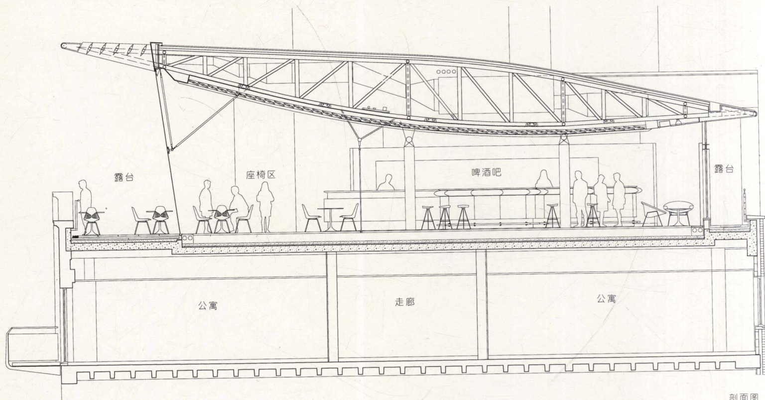
剖面图
