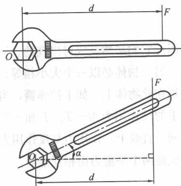
图 1-3 力矩
