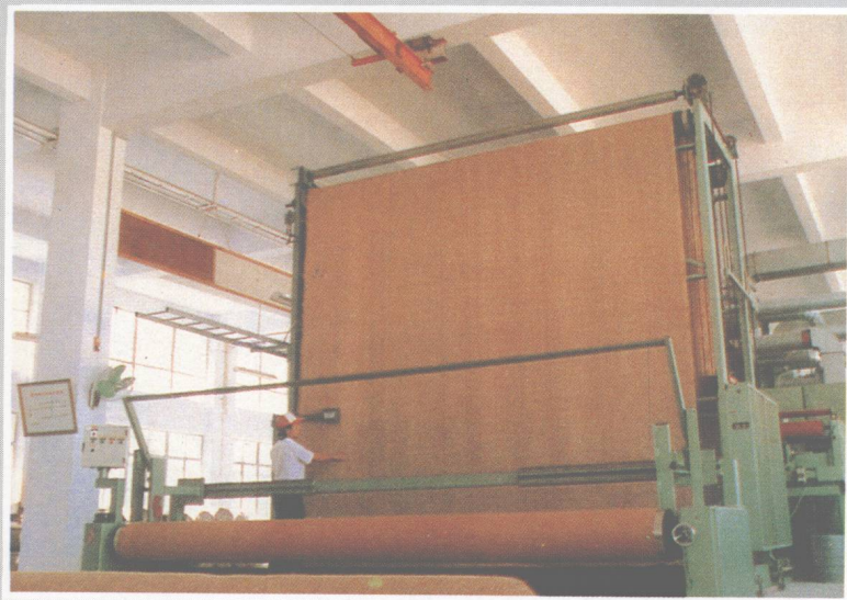
引进丹麦地毯背面涂层生产线
