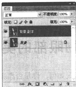
图1-3 复制图层
