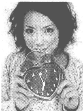
图1-28 修复右眼
