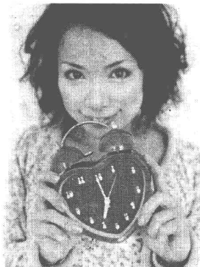
图1-27 打开素材
