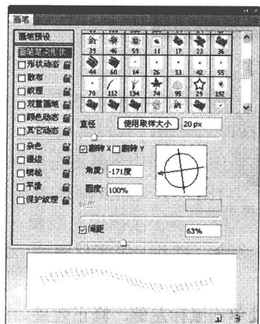
图1-23 调整参数
