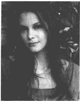
图1-1 消除黑眼圈
