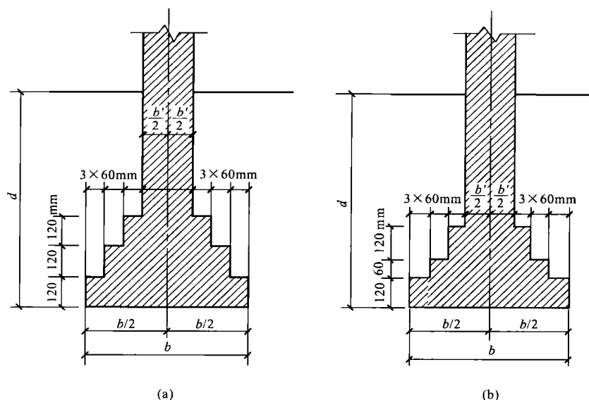
图 1-1 砖基础
