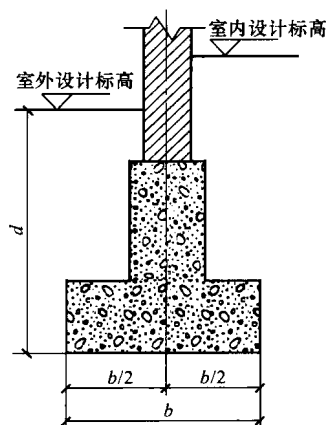
图 1-4 毛石混凝土基础
