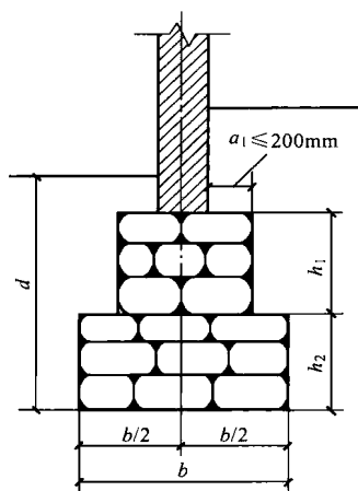
图 1-2 毛石基础
