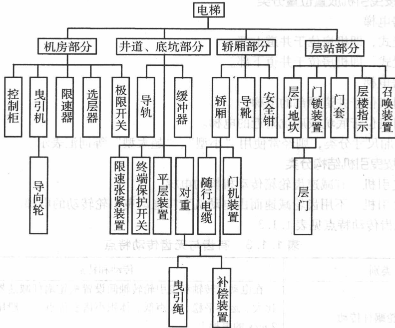
图 1.1.5 电梯的基本组成
