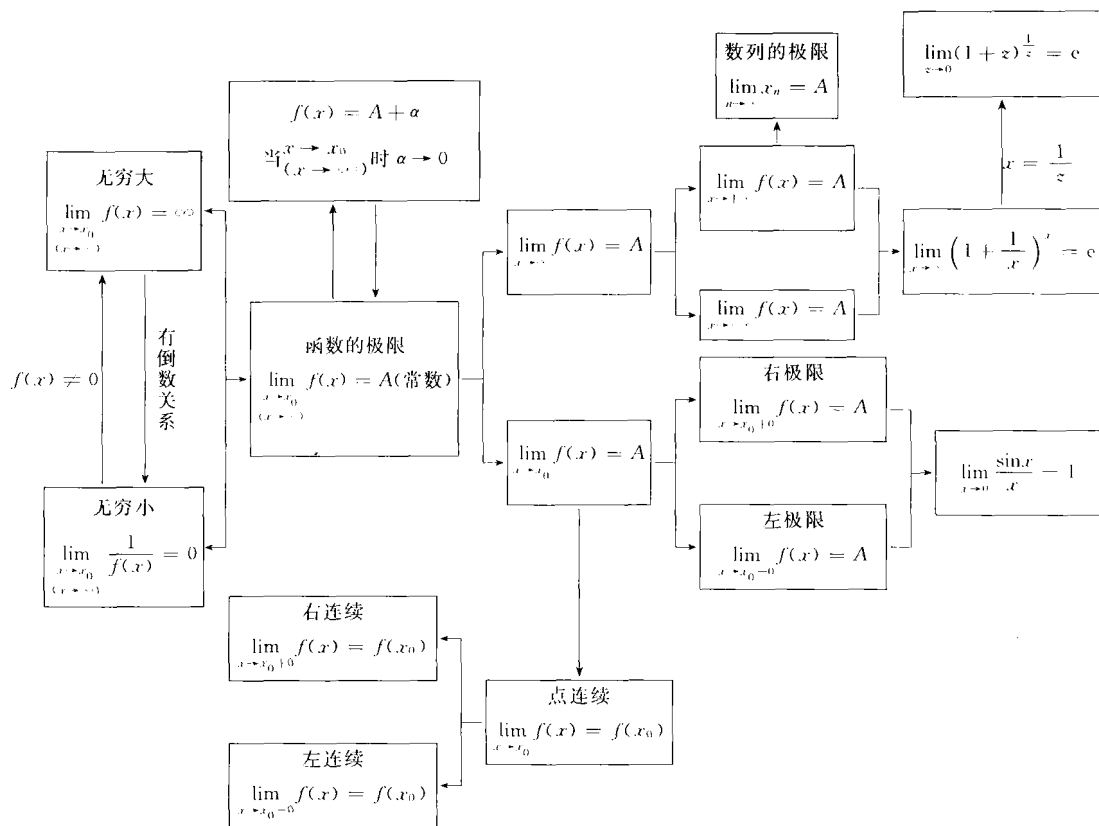
图 1-1 函数的极限及其引申概念之间的关系
