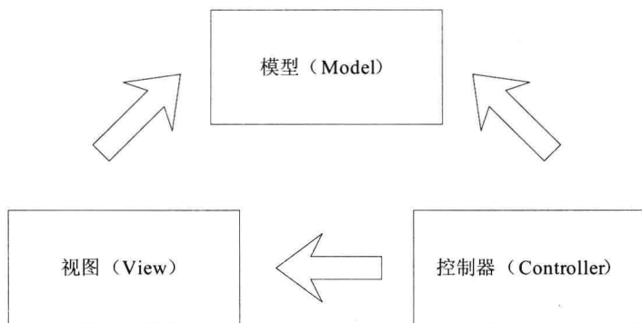
图 1-1 MVC 示意图
