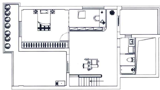
● 二层平面图
