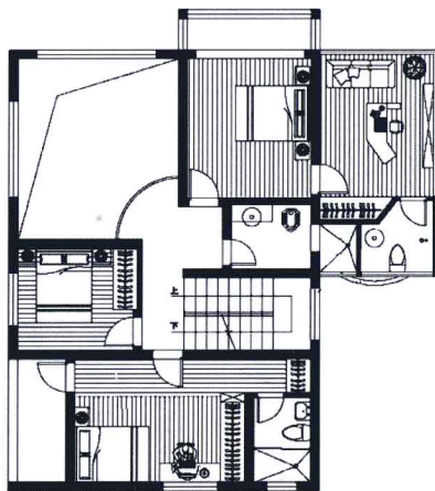
● 二层平面图
