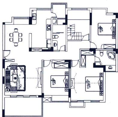
● 一层平面图
