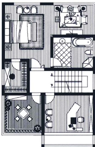
● 三层平面图
