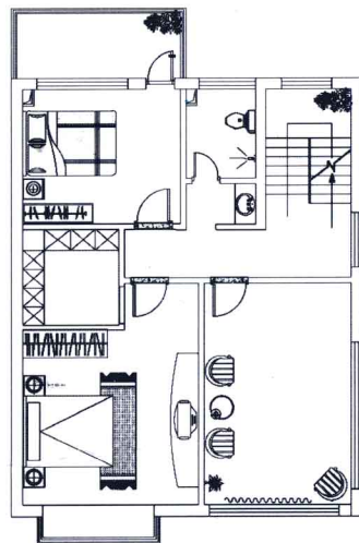
● 二层平面图
