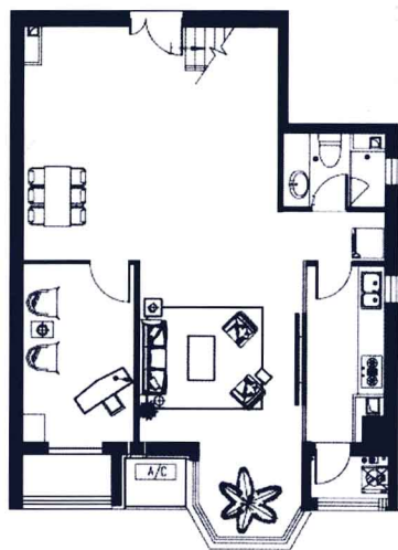
● 一层平面图
