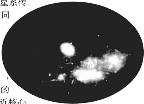
飞马座星系团里有一个环状星系
