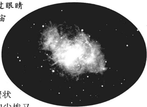
蟹状星云是一颗恒星的墓地
