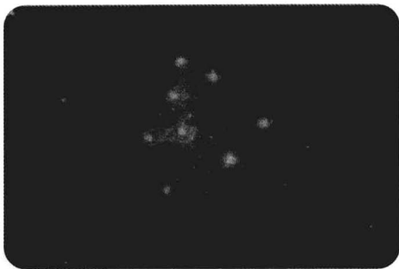
昴星团是一群年轻的恒星
