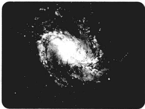
漩涡 涡状星云像 太空中的龙 卷风
